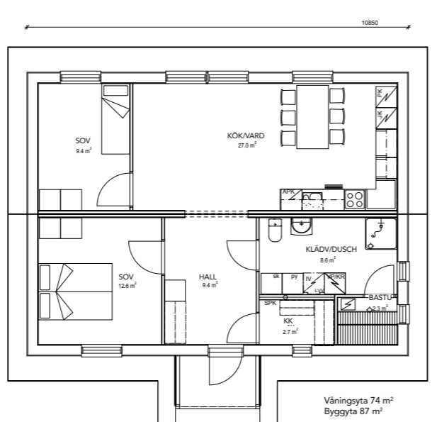
MODELL 74B (våningsyta 74 m 2 )
