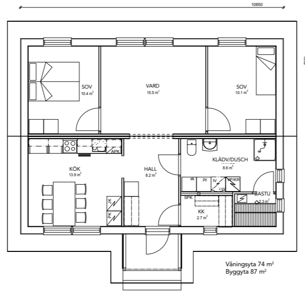
MODELL 74A (våningsyta 74 m 2 )
