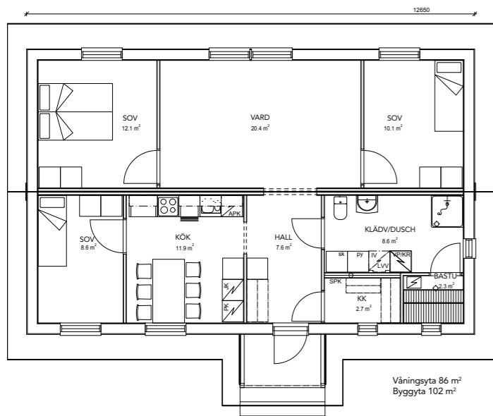
MODELL 86A (våningsyta 86 m 2 )
