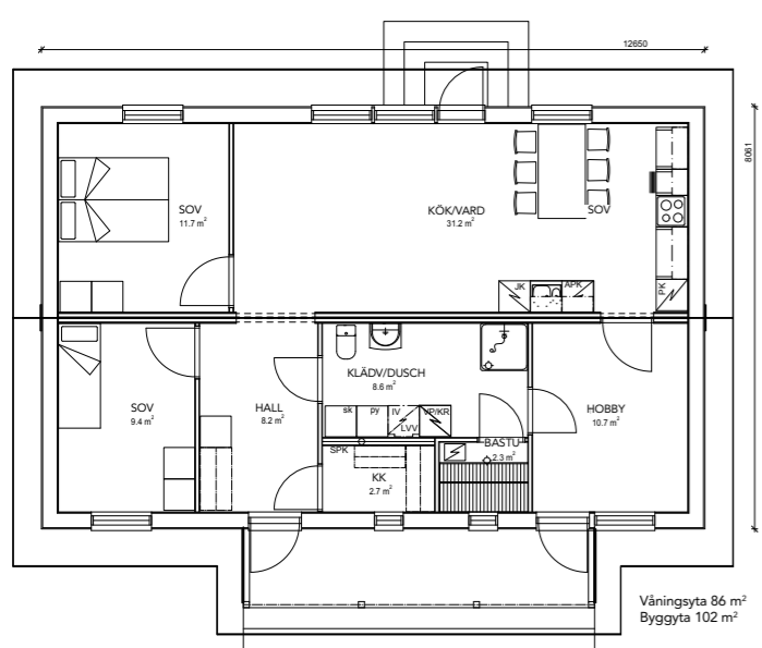
MODELL 86B (våningsyta 86 m 2 )
